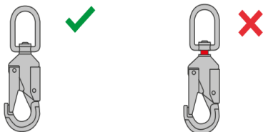
Obrázek 1 Indikátor zatížení
